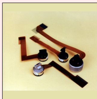
54. Głowice małogabarytowe do drukarek 1986 - 2003
