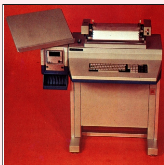
35. Minikomputer MERA-100 1980-1988
