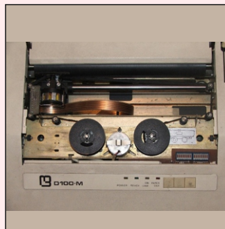
48. Drukarka mozaikowa małogabarytowa D-100 1986-1990
